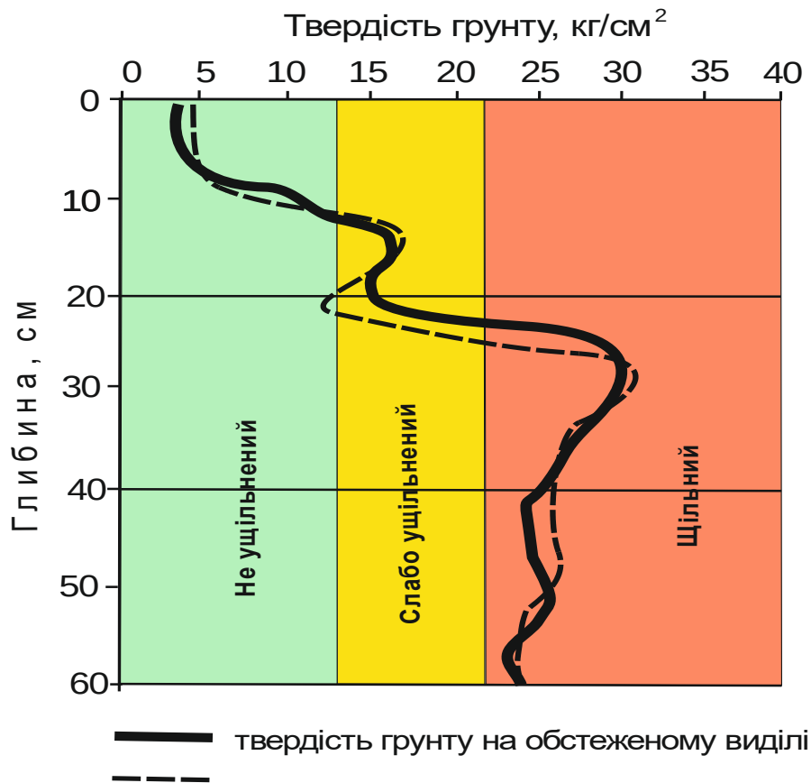
Рис. 7. Крива твердості ґрунту після проведених рубок головного користування берези повислої (квартал 15, виділ 30 Новоставського лісництва) у порівнянні з контролем
